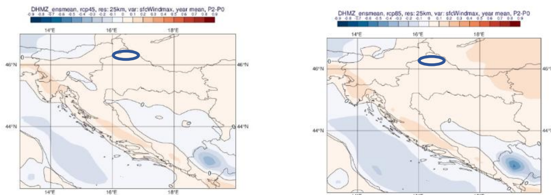
Slika 9 Promjena srednje godišnje maksimalne brzine vjetra na 10 m (m/s) u odnosu na referentno razdoblje 1971.-2000. godine u srednjaku ansambla iz četiri integracije RegCM modelom. Gore: za razdoblje 2011.-2040. godine; dolje: za razdoblje 2041.-2070. godine. Lijevo: scenarij RCP4.5; desno: scenarij RCP8.5.
