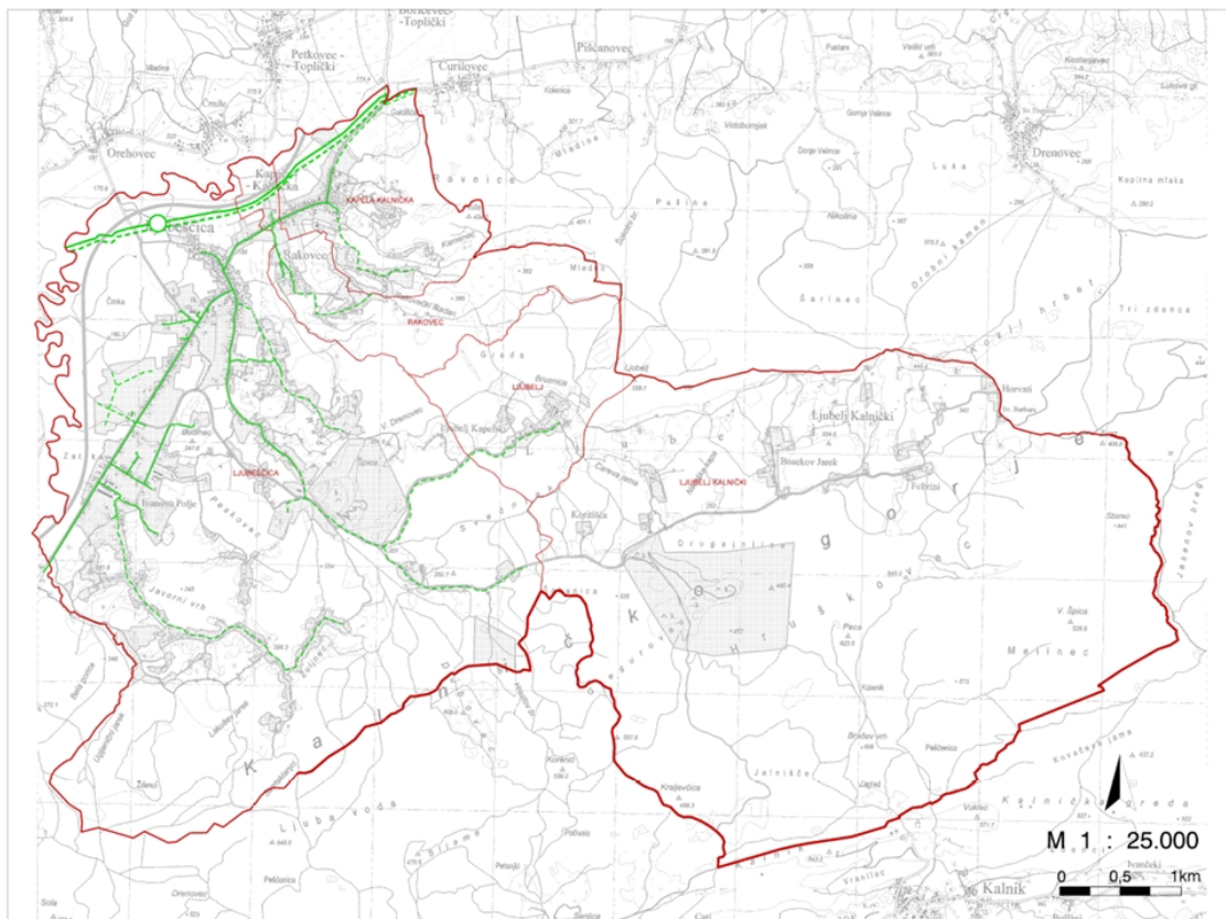
Slika 10. Prikaz infrastrukture plinovoda na području Općine Ljubešćica
