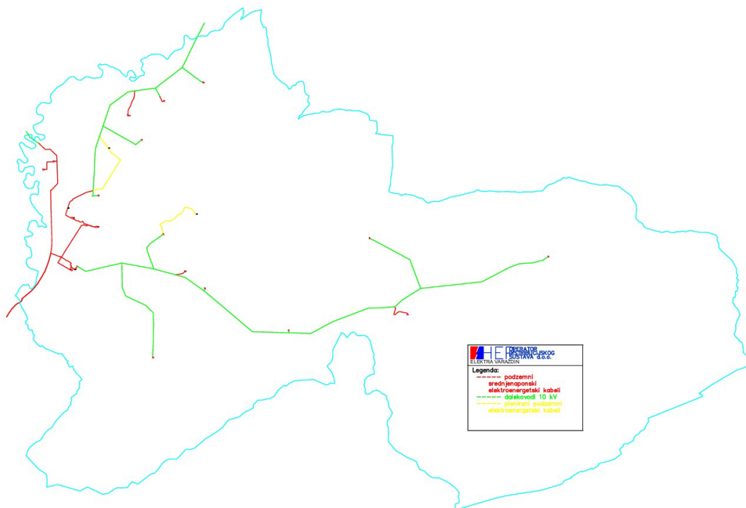
Kartogram 6. Elektroenergetska mreža na području Općine Ljubešćica
