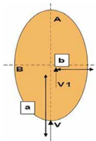
Tablica 23. Prikaz brzine širenja požara u odnosu na brzinu vjetra
