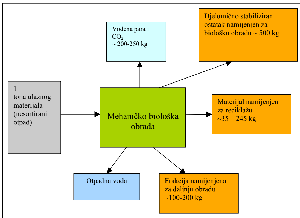
Slika 3: Shematski prikaz tipičnog sustava mehaničko biološke obrade otpada
