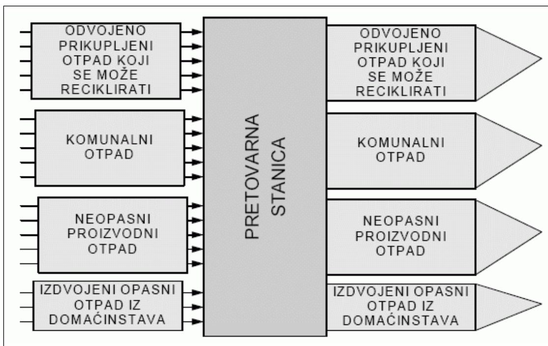
Slika 4. Tok otpada kroz pretovarnu stanicu
