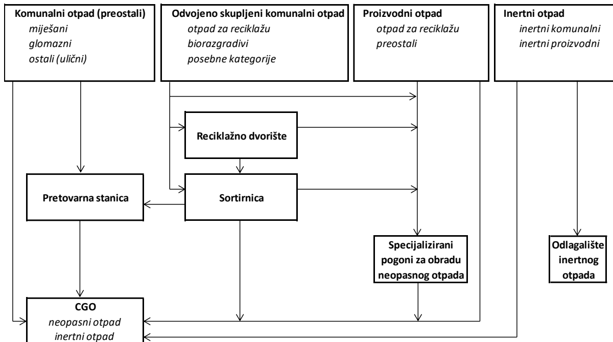
Slika 2.2/1 - Shema gospodarenja neopasnim i inertnim otpadom (izvor: IPZ Uniprojekt TERRA)
