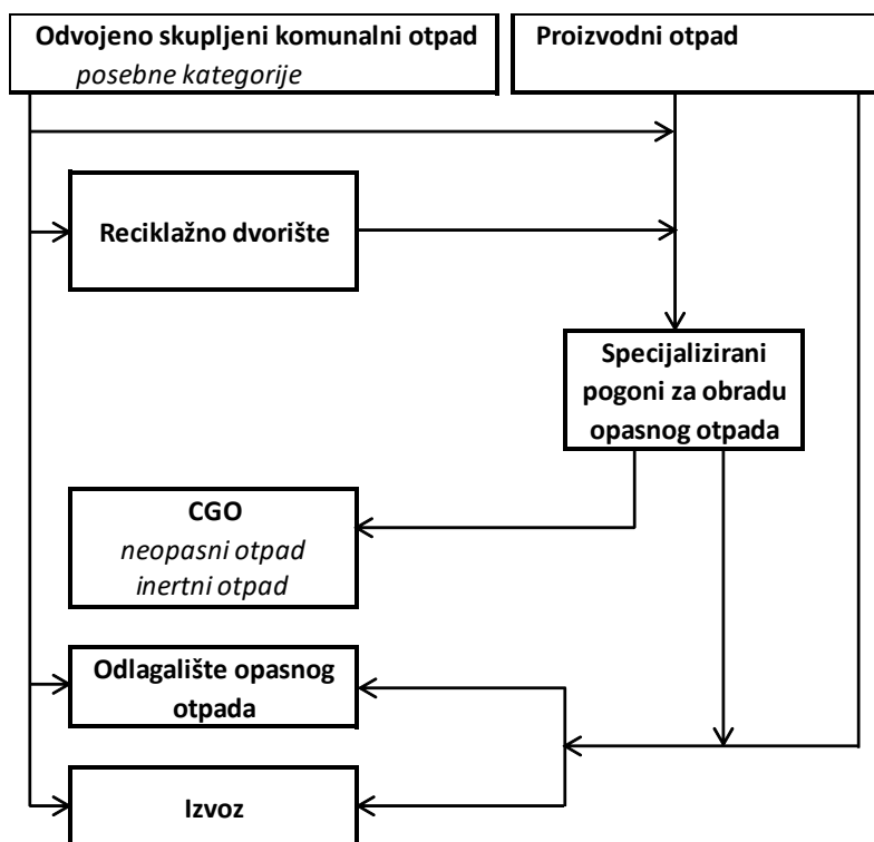
Slika 2.2/2 - Shema gospodarenja opasnim otpadom (izvor: IPZ Uniprojekt TERRA)
