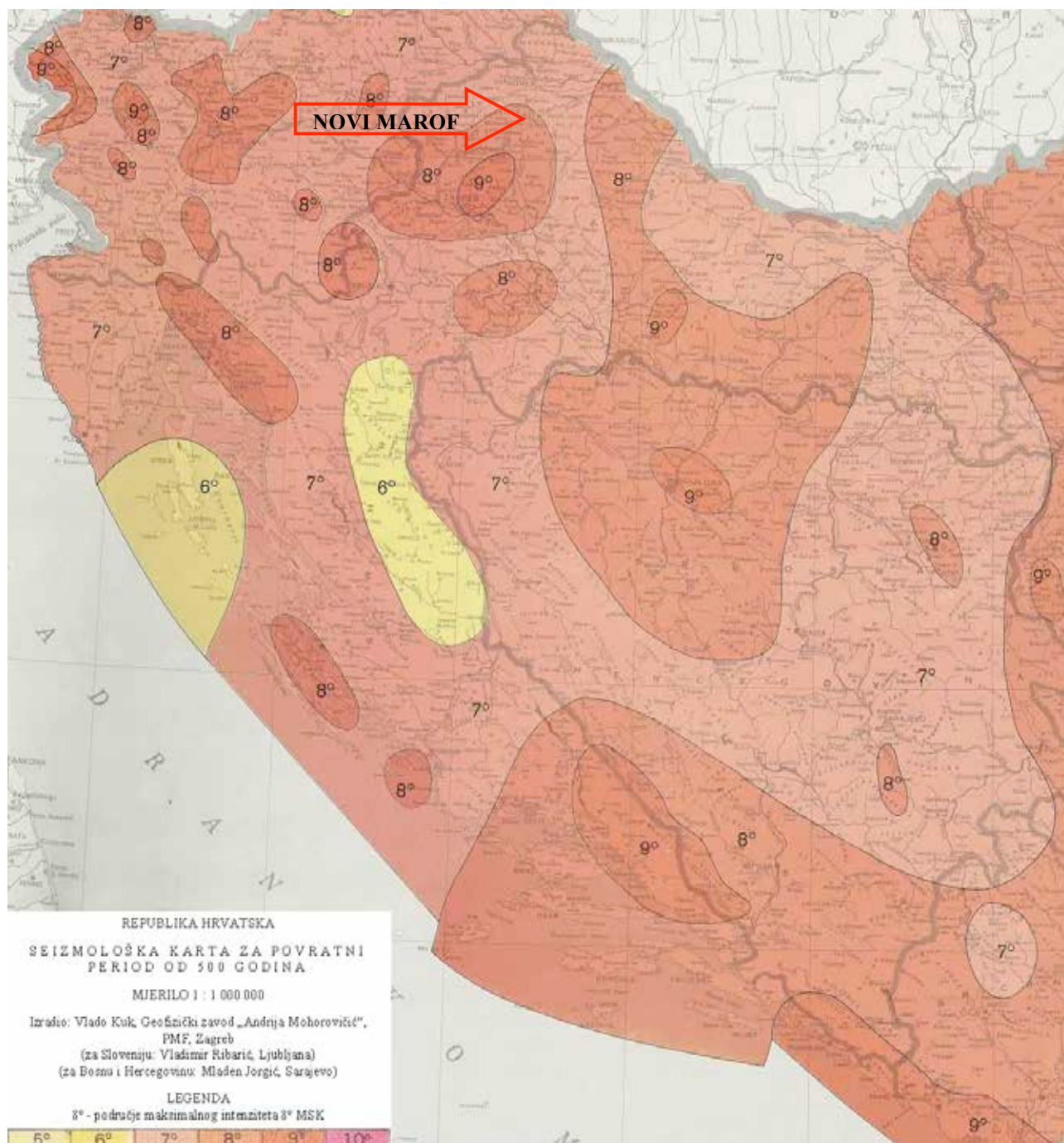
Slika 4: Seizmološka karta za povratni period T=500 godina Izvor PMF, Zagreb
