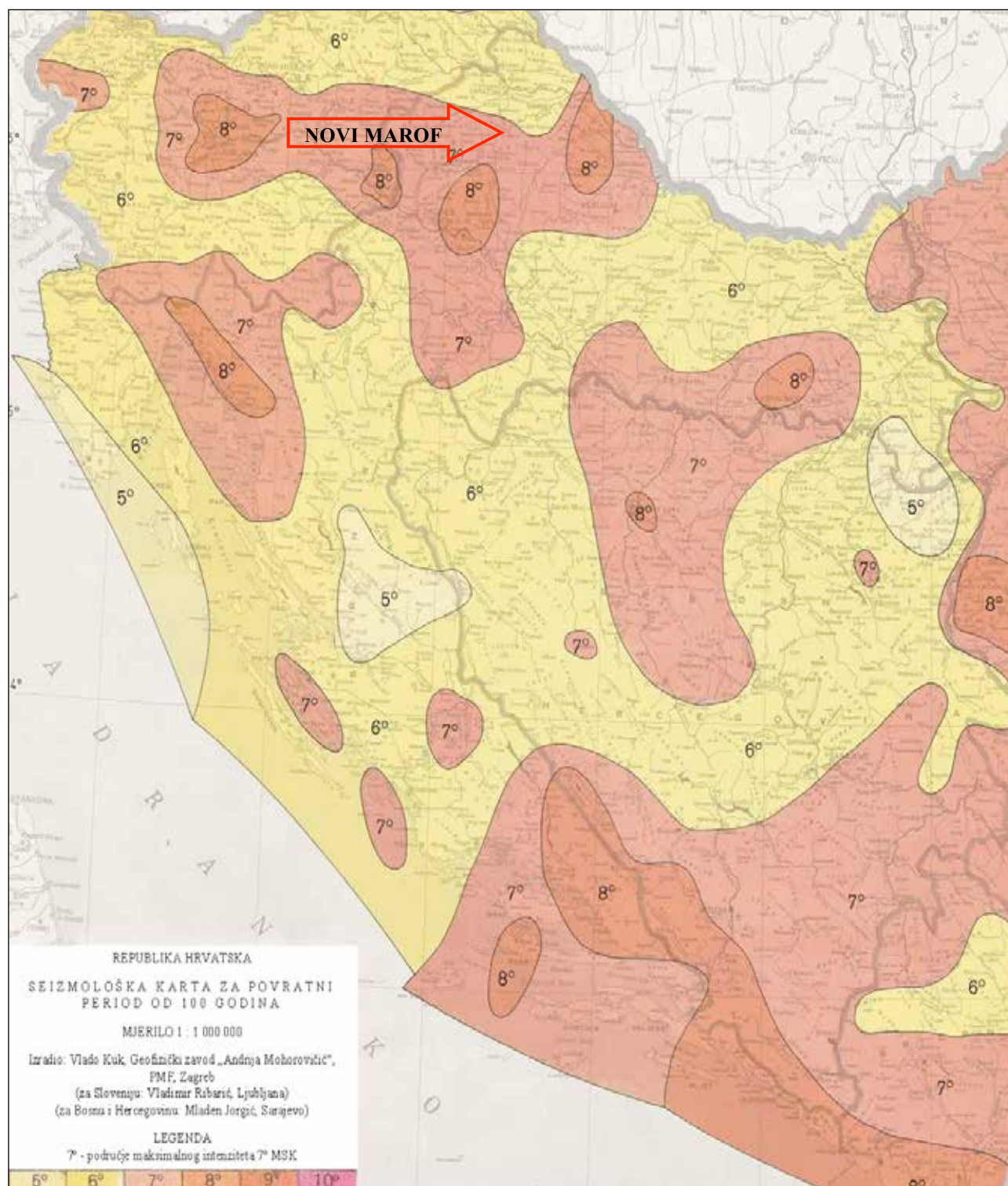
Slika 2: Seizmološka karta za povratni period T=100 godina Izvor PMF, Zagreb
