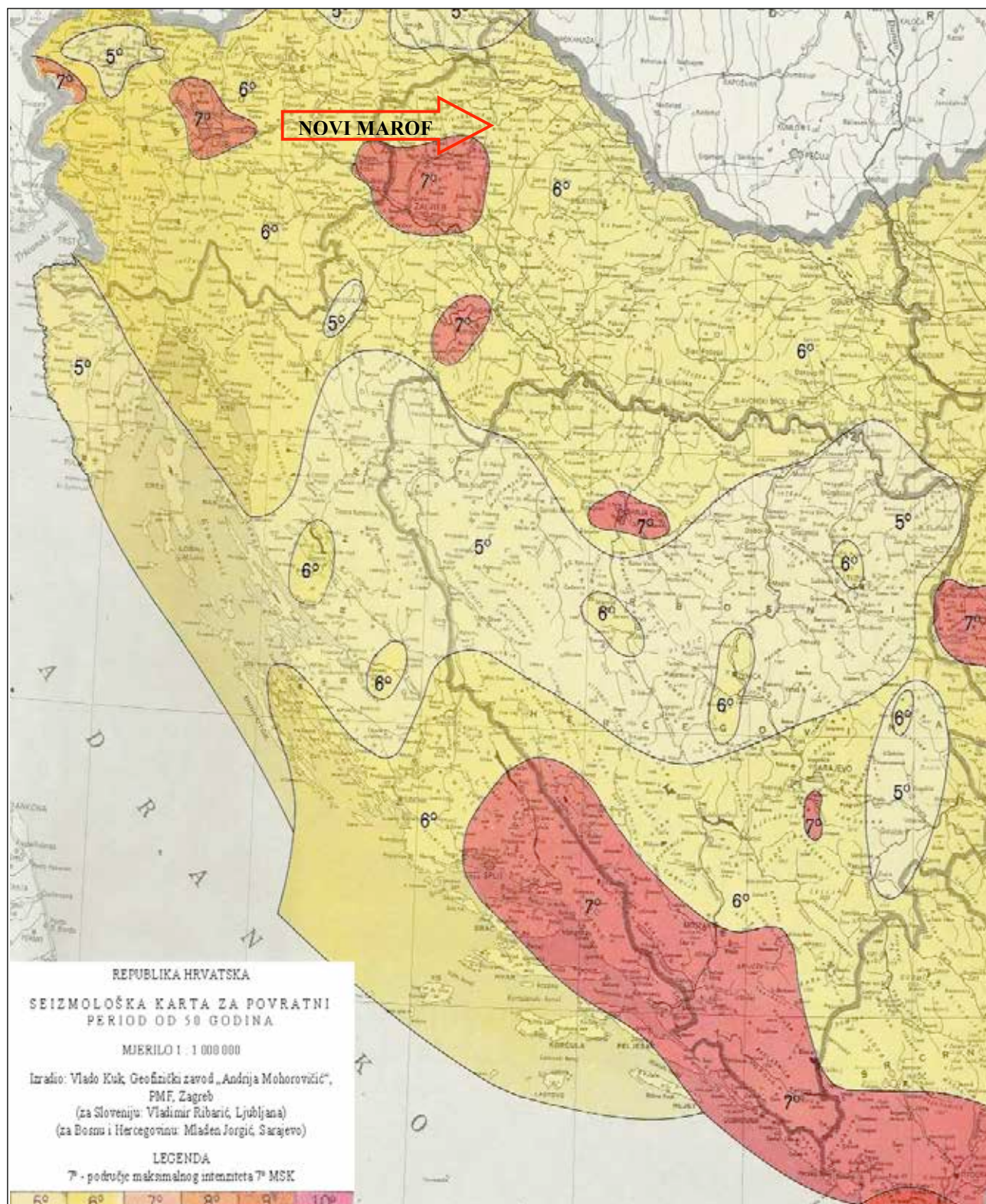
Slika 1: Seizmološka karta za povratni period T=50 godina Izvor PMF, Zagreb
