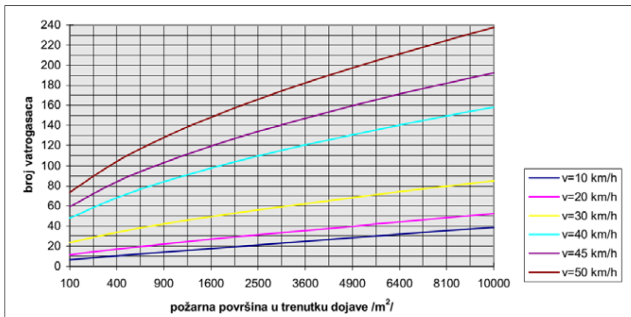
Slika 7: Grafički prikaz potrebnog broja vatrogasaca N_v za gašenje požara otvorenih prostora u periodu intervencije t=15 min, pri brzini vjetra v=10-50 km/h
