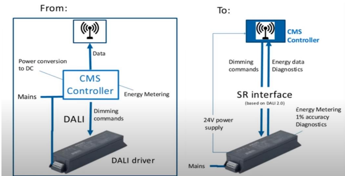
Slika 8 Prednosti SR drivera za sustav upravljanja
