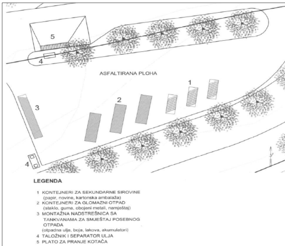
Slika 2. Shematski prikaz reciklažnog dvorišta
