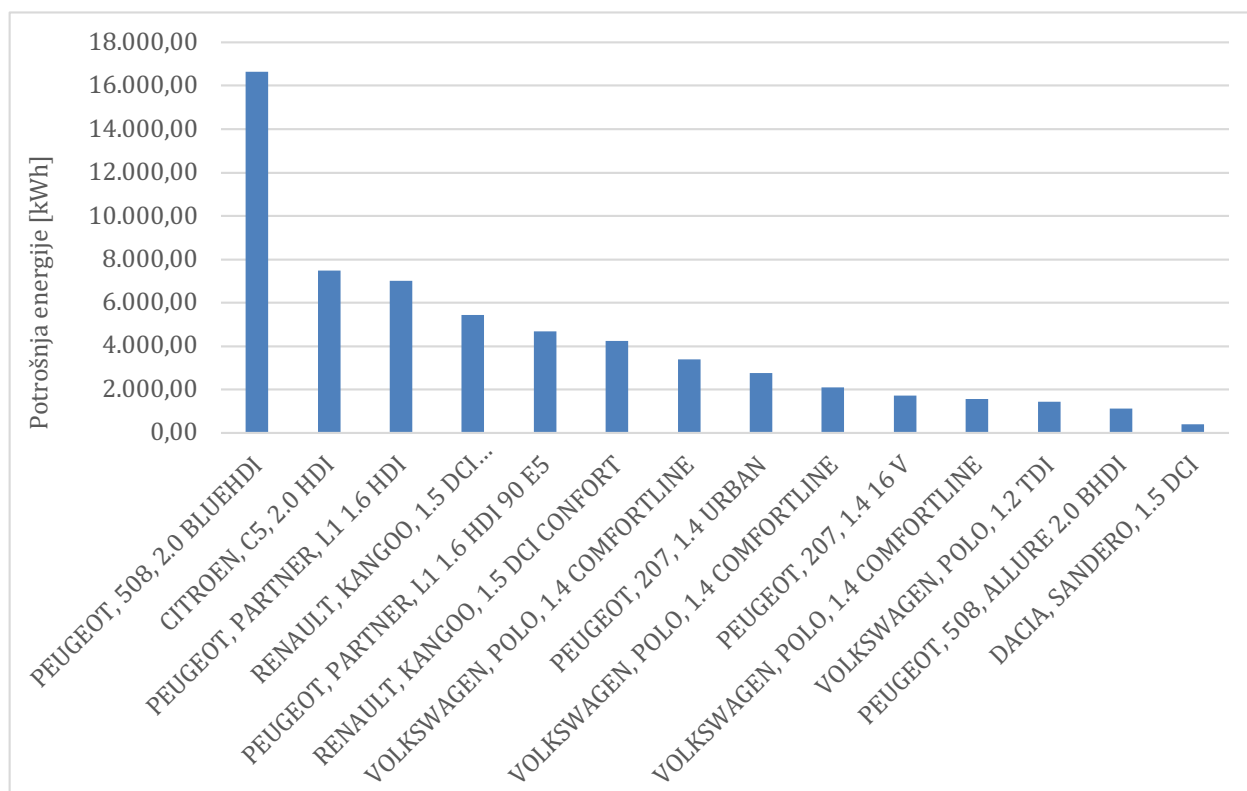
Slika 3 Usporedna potrošnja energije po vozilima
