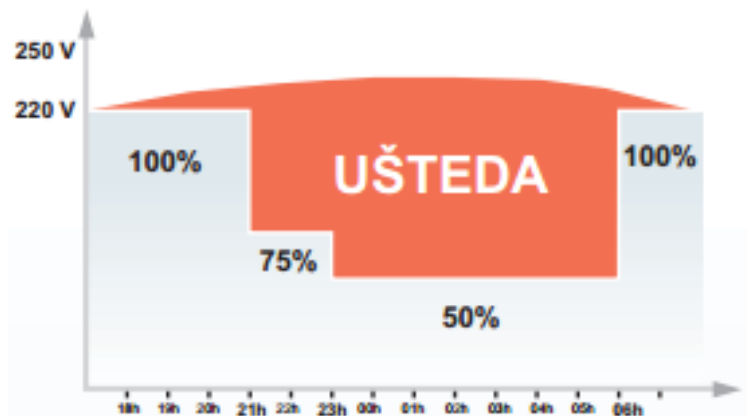
Slika 6 Grafički prikaz ušteta ostvarenih regulatorom
